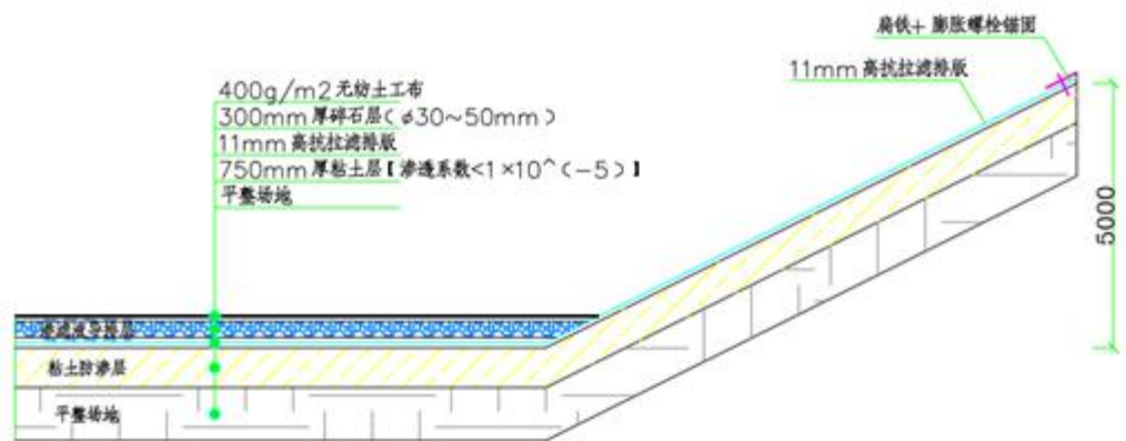
图 2.7.3-1 防渗层结构图
