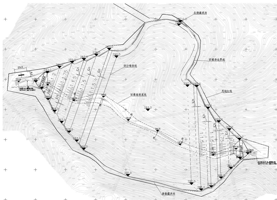
图 2.7-1 回填区域总体布局图
