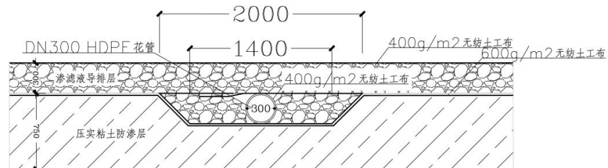
图 2.7.4-1 淋溶水导排盲沟
