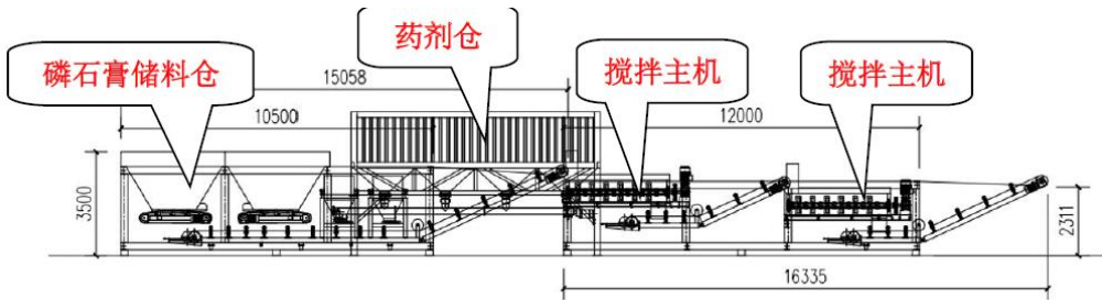
图 2.3.3-1 无害化处理设备布置图
