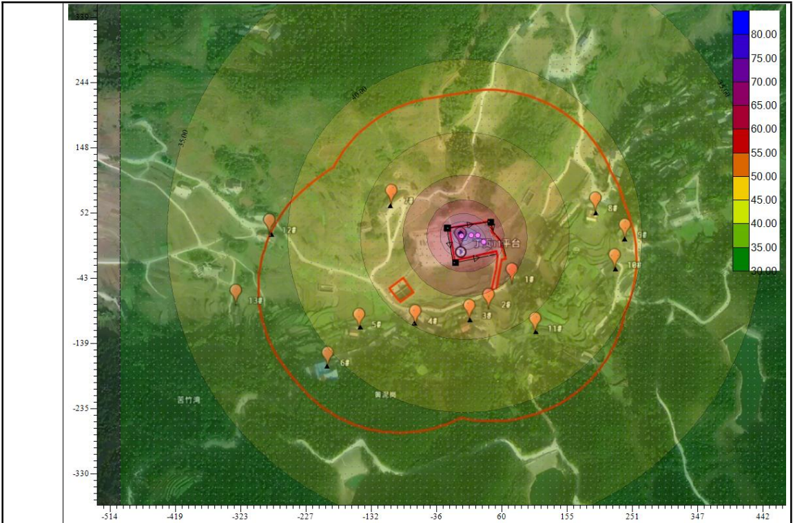
图 4-1 项目施工期噪声预测结果图
