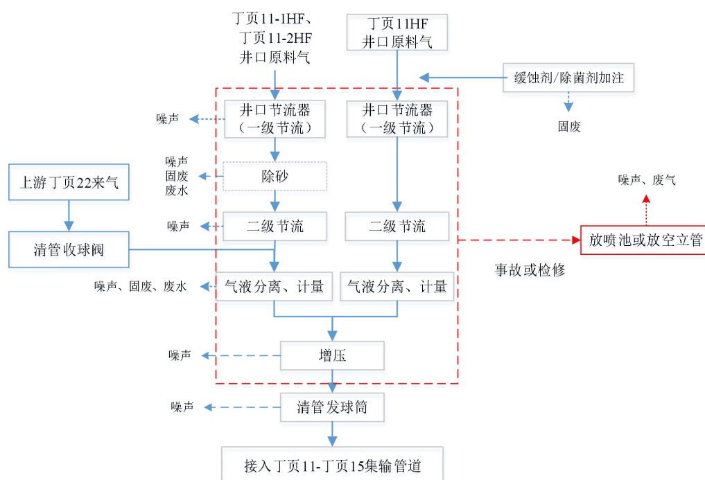
图 2.13-1 丁页 11 平台工艺流程及产排污环节图
