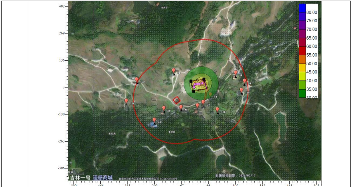
图 4.2-1 噪声预测结果
