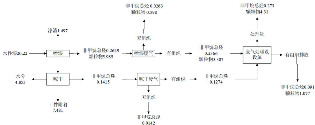
图 2.1-1 本项目水性漆非甲烷总烃平衡图 单位：t/a
