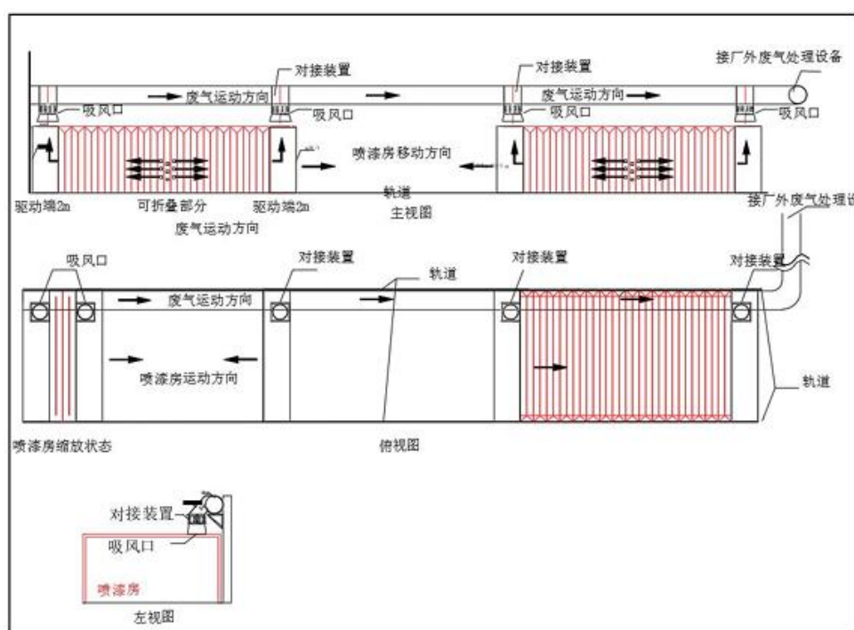
图 2.2-3 移动喷漆房示意图
