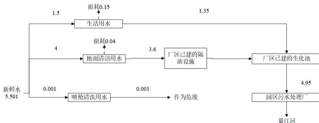
图 2.1-2 项目水平衡图（日最大排水量 m 3 /d）
